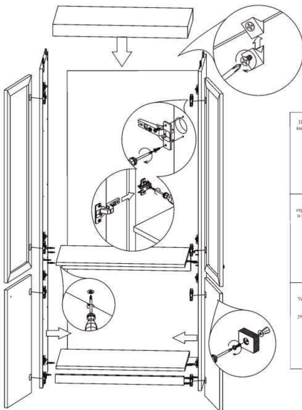
Установка полок с помощью усиленных эксцентриков
